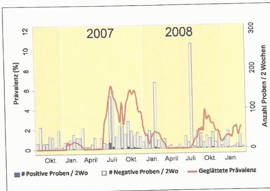
Abbildung 3: Zeitlicher Verlauf der LPAI-positiven Tupferproben.
